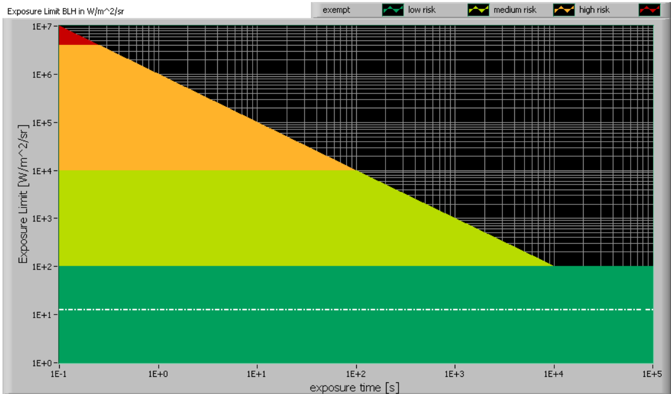
Das Niveau des blauen Lichtes dieser Lampe, und die Zusammenhang mit dem Grenzwert und die unterschiedliche Einstufung Bereichen.
