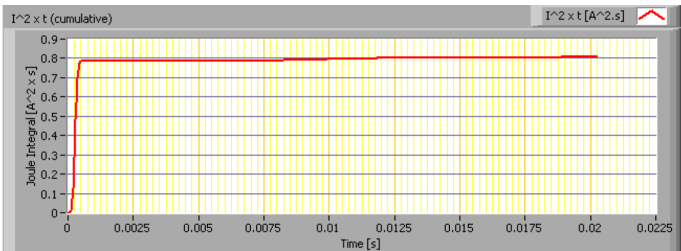
De waarde I^2 \cdot \Delta t uitgezet tegen tijd, voor de eerste 10 ms.
