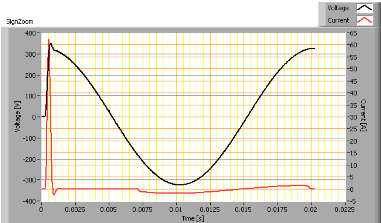
Eerste cyclus van de inschakelstroom.
