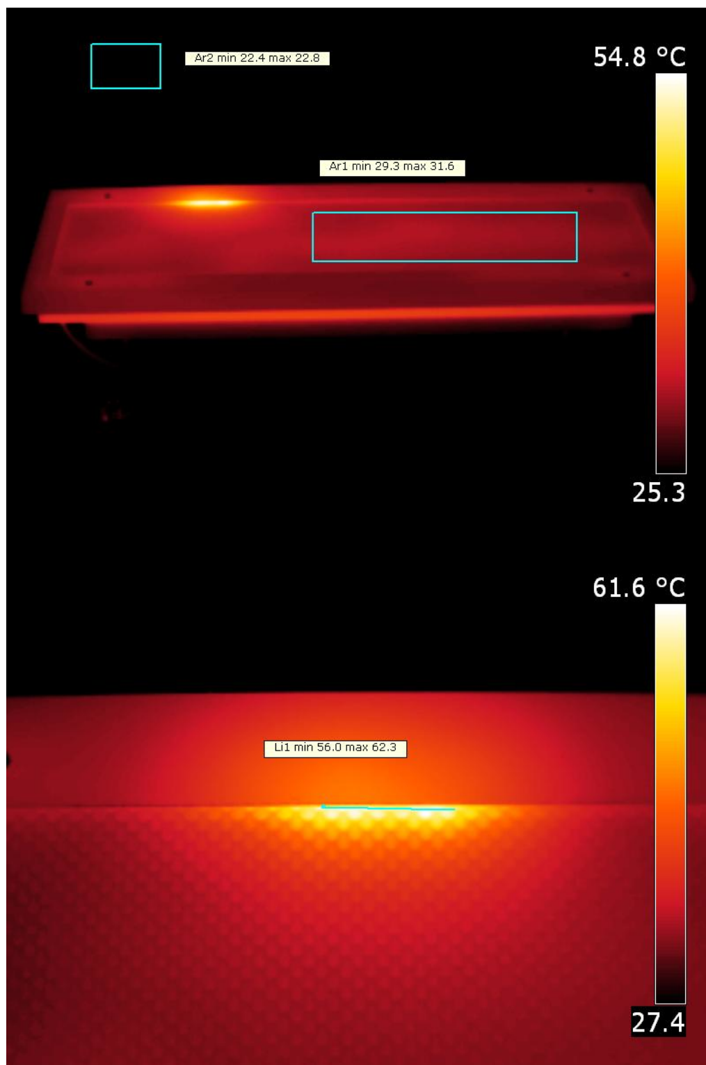
Temperatuursmeting vooraanzicht
