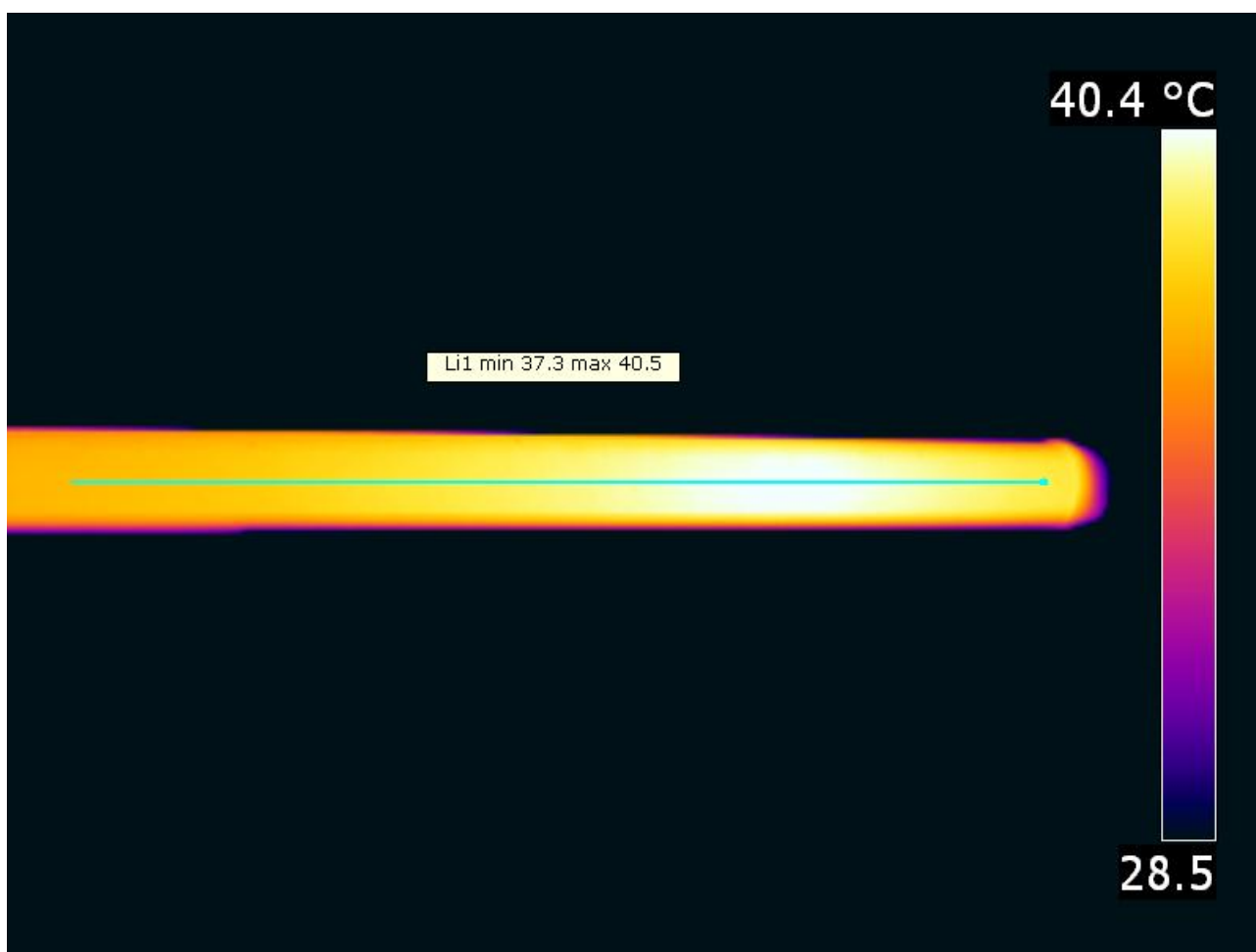
Temperatuursplaatjes van het metalen gedeelte van de buis.
