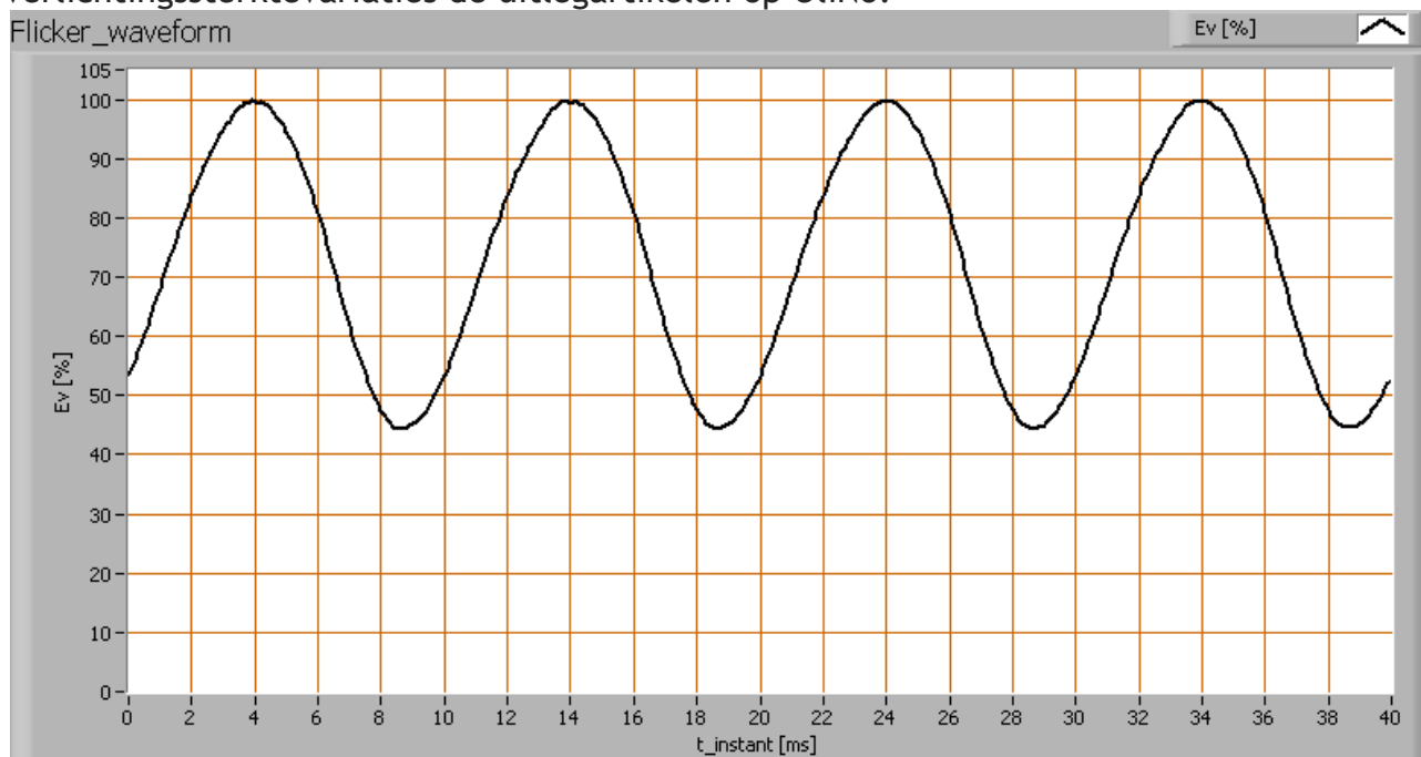
De mate van snelle verlichtingssterktevariati s van het licht van de lamp
