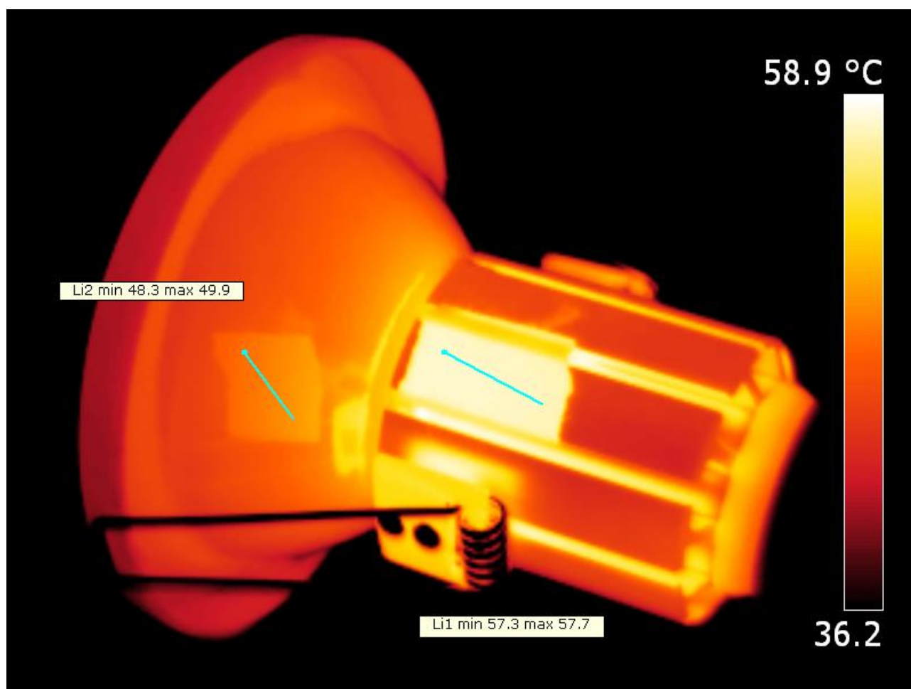
Temperaturbilder.
