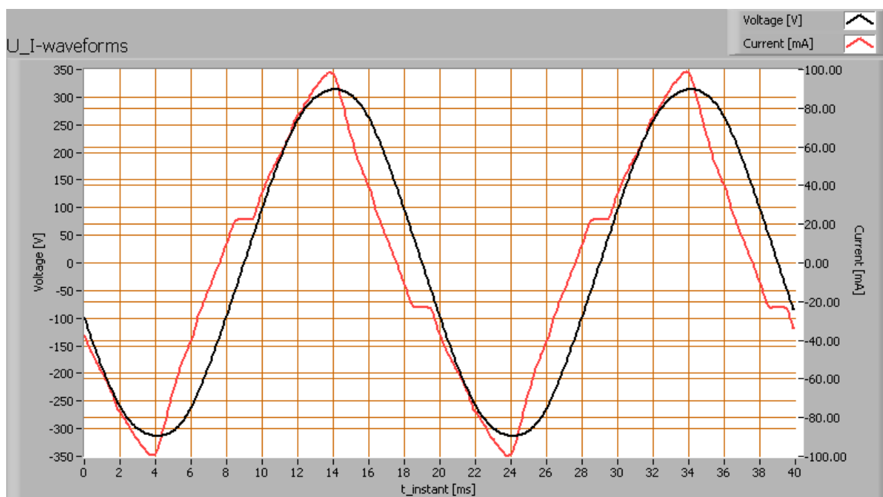
Spannungsverlauf an der Lampe und Stromverlauf durch die Lampe
