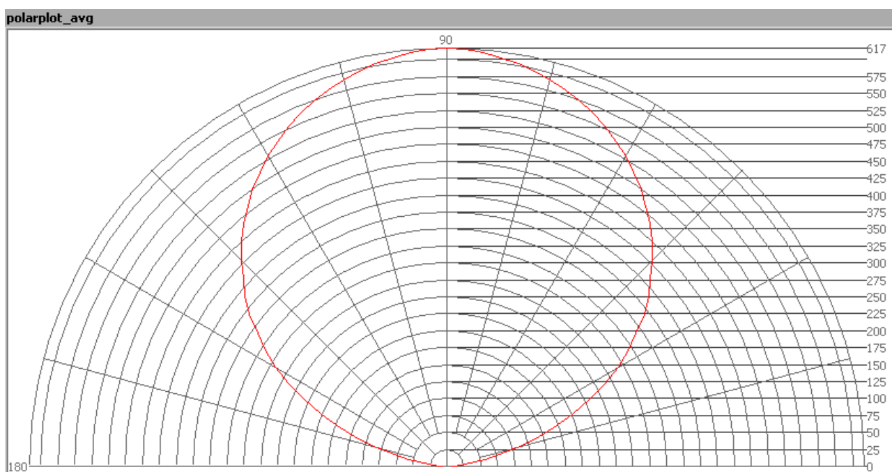
Das Strahlungsdiagramm der Lampe.
