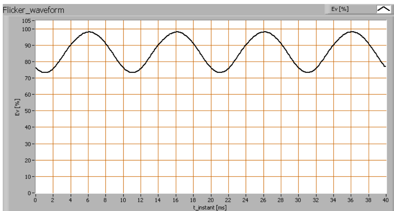
Mesure des variations d'intensité d'éclairement rapides de la lumière de la lampe
