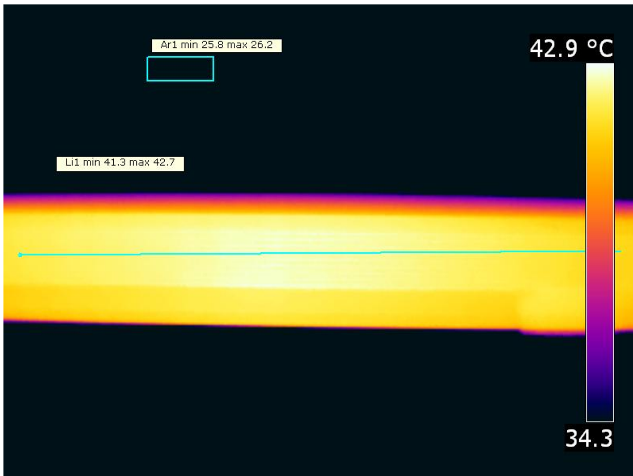
Image de température. L'émissivité de aluminium est de 0.92.
